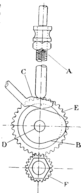
FIG. 30. VALVE CAM ACTION
