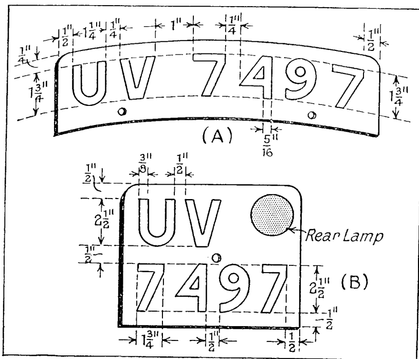
FIG. 21. NUMBER PLATE DIMENSIONS
