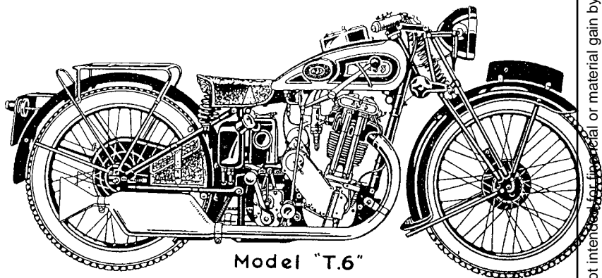
FIG. 9. THE 3.49 H.P. O.H.V. DE LUXE MODEL T6 (TWO PORT)
